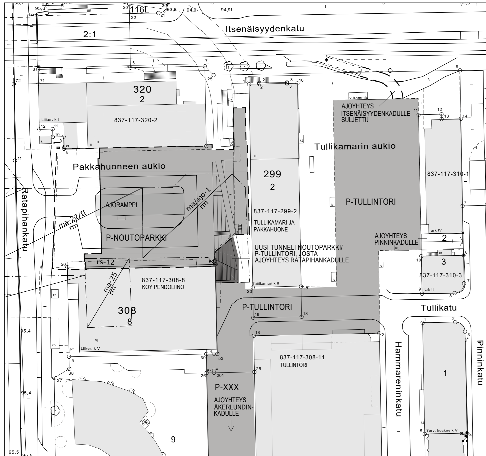
SUUNNITELMA N2000-JÄRJESTELMÄSSÄ.
